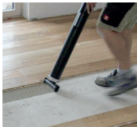
Stěna nebo hrana parkety slouží jako boční svodidlo pro roznášecí hlavu.
